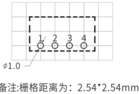
3)建议印刷版图
