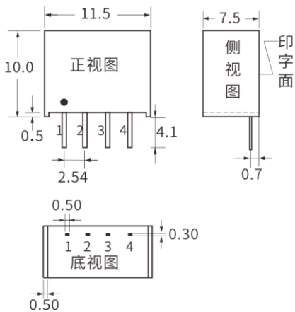
1)外观尺寸(单位: mm,公差: xx ±0.25)
